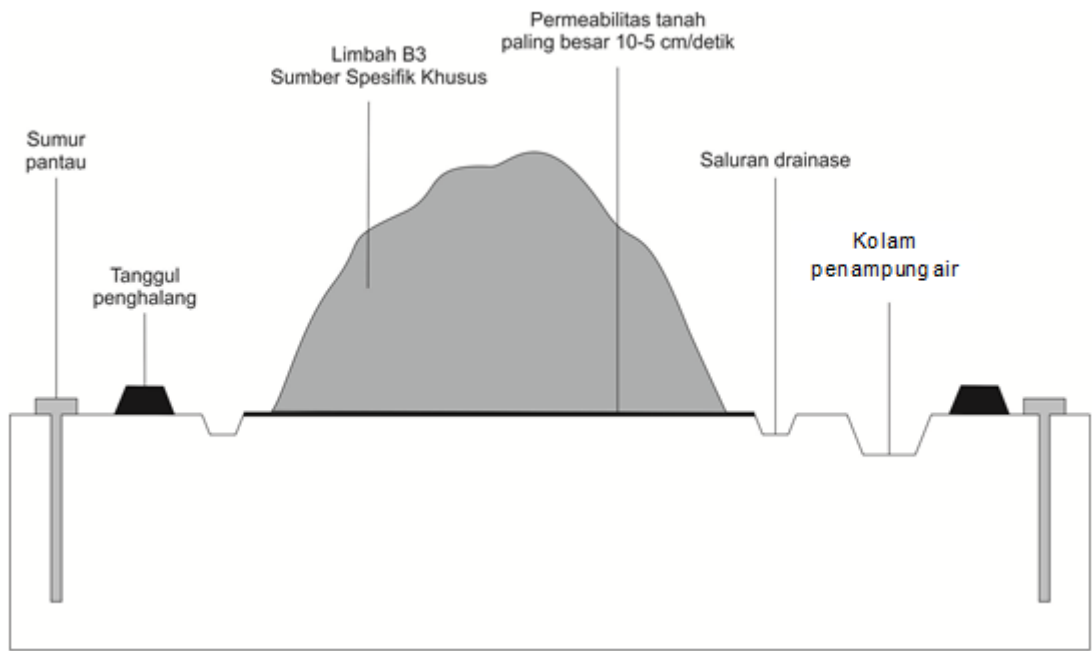
Gambar 5. Contoh Rancang Bangun fasilitas Penyimpanan Limbah B3 berupa tempat tumpukan Limbah B3 ( waste pile )
